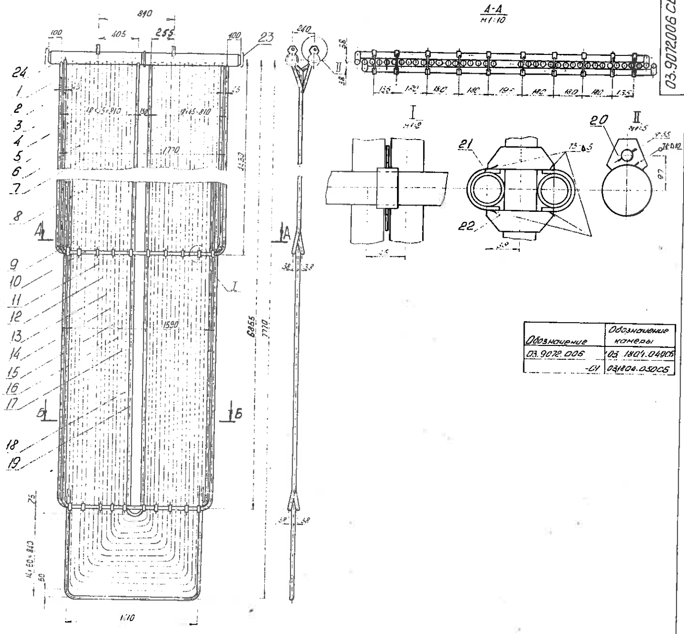
Схема сборки 1-го ряда по черт. 03.9072.006
