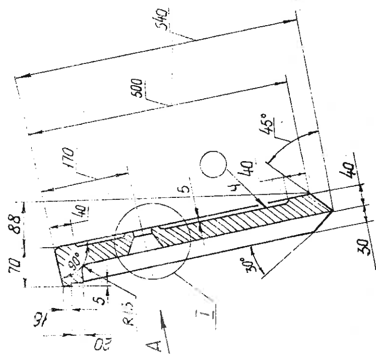
Вид А повернуто М1:2
